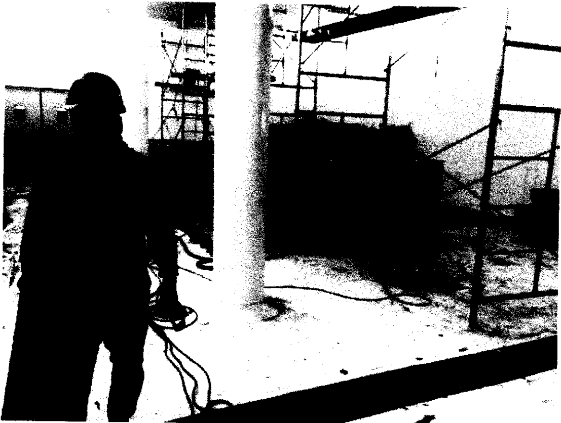
Fotografía N°09: Instalación de viga de acero para grúa móvil sobre poza de acero.
